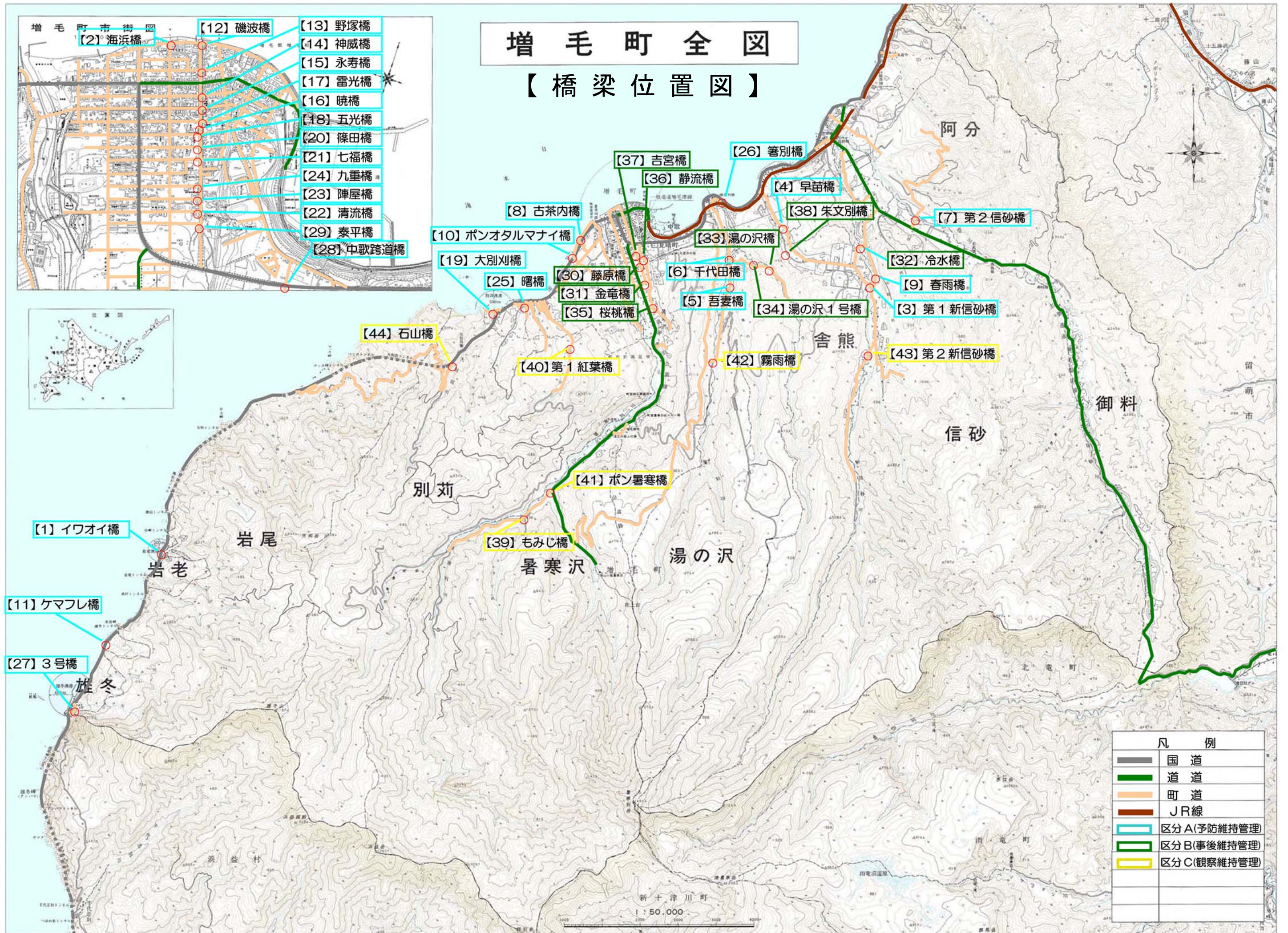
図 2.1 対象橋梁位置図
